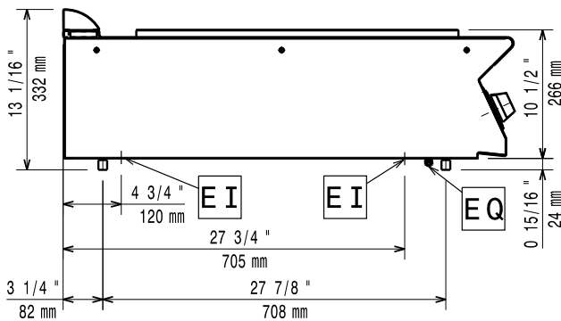
Zij aanzicht
